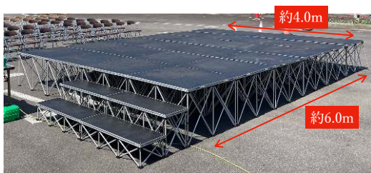
主催者側準備 屋外特設ステージ（約6.0m×4.0m、高さ約1.0m）
